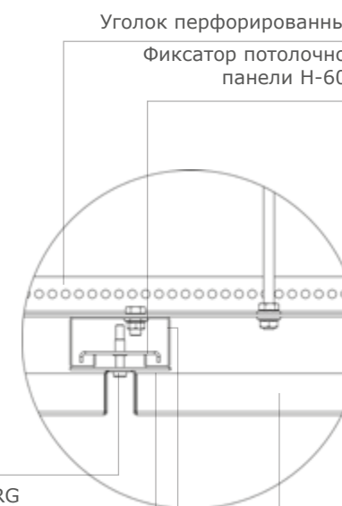
ВИД В. ТИПОВОЙ ВИД НА ПОДСИСТЕМУ
