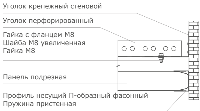
УЗЕЛ КРЕПЛЕНИЯ СТЕНОВОЙ ПАНЕЛИ
