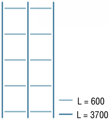
СХЕМА МОНТАЖА
